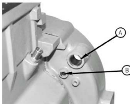
Контрольное отверстие установочной метки угла поворота коленвала в картере маховика двигателя
