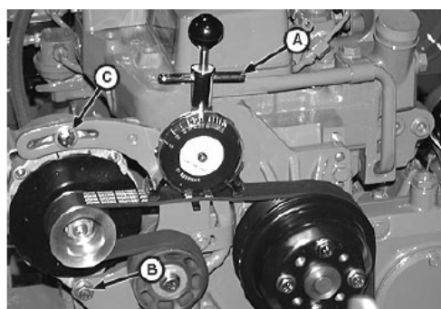
Проверка натяжения ремня
