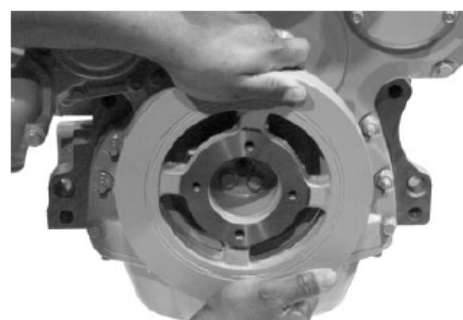
Взяться за демпфер крутильных колебаний
