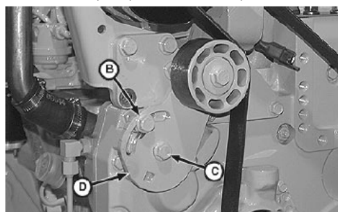
Регулировка натяжения ремня
