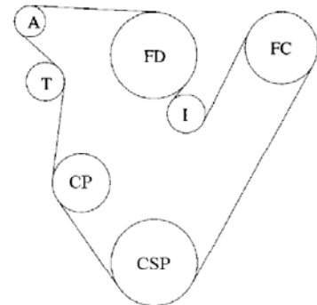
402 мм. Высота расположения оси вентилятора со шкивом компрессора кондиционера *
