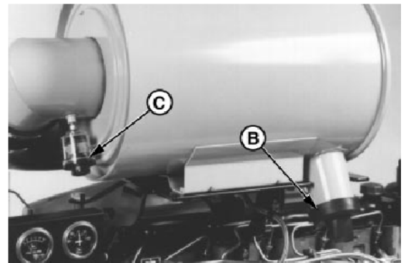
Клапан сброса пыли и индикатор засоренности
