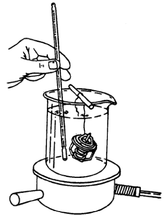
Проверка температуры открытия термостатов
